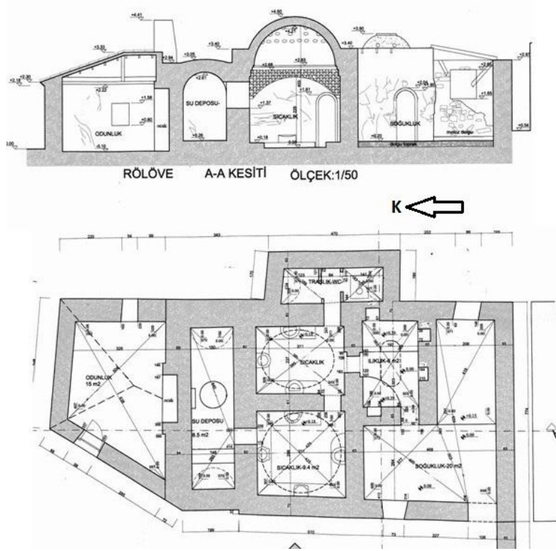
Şek.5. Büyük Anafarta Hamamı, plan ve kesit (Mim. B. Köylü'nün izniyle)
