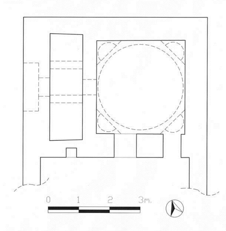
Şek.4- Yenişehir (Burhan) hamam planı (aou)
